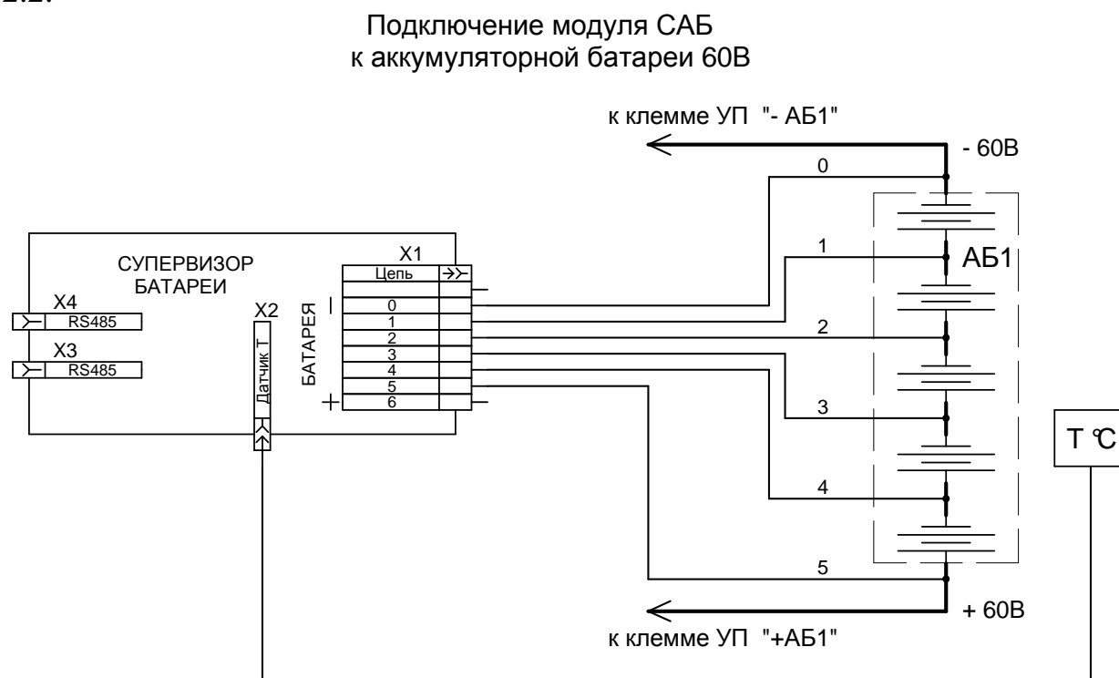
Рисунок 2.2 – Схематическое изображение подключения модуля САБ для поэлементного контроля АБ
